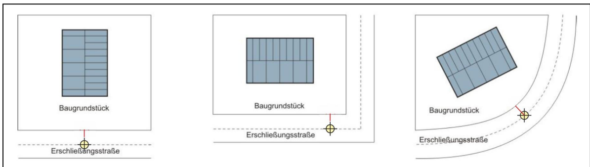
Abb. 7: Prinzipskizze maßgebender unterer Bezugspunkt
