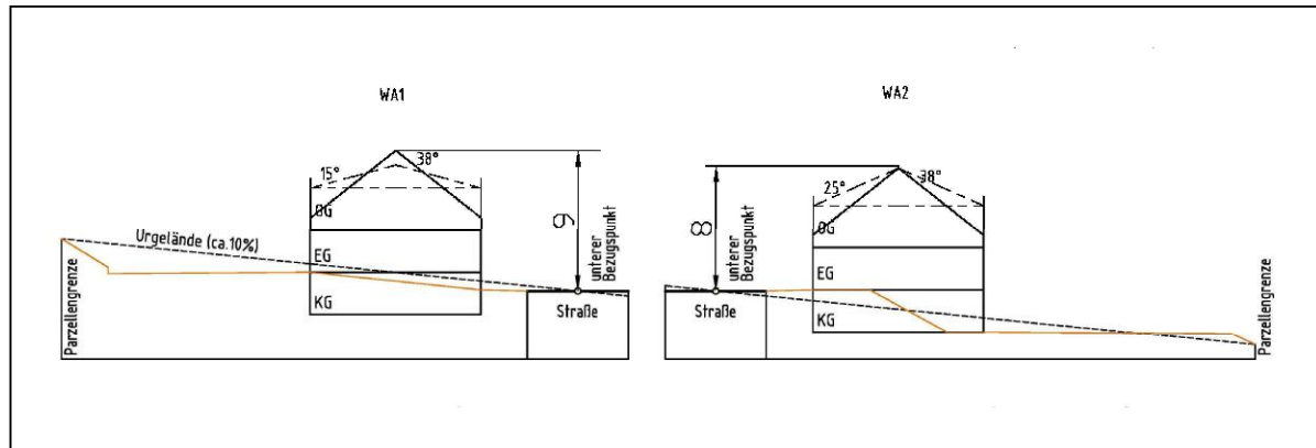
Abb. 7: Schemaschnitt mit Höhen, Bezugspunkten und möglicher Geländegestaltung – unmaßstäblich
